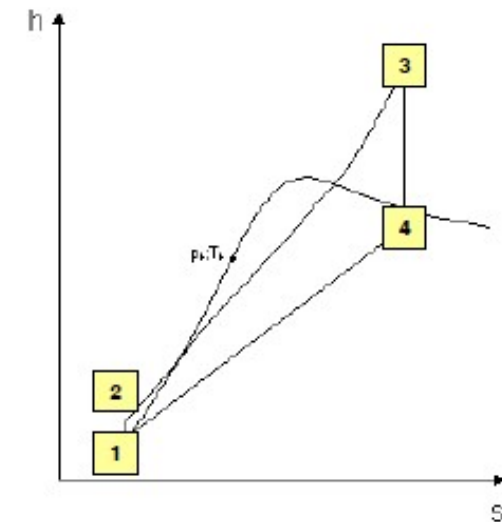
h-s-Diagramm
