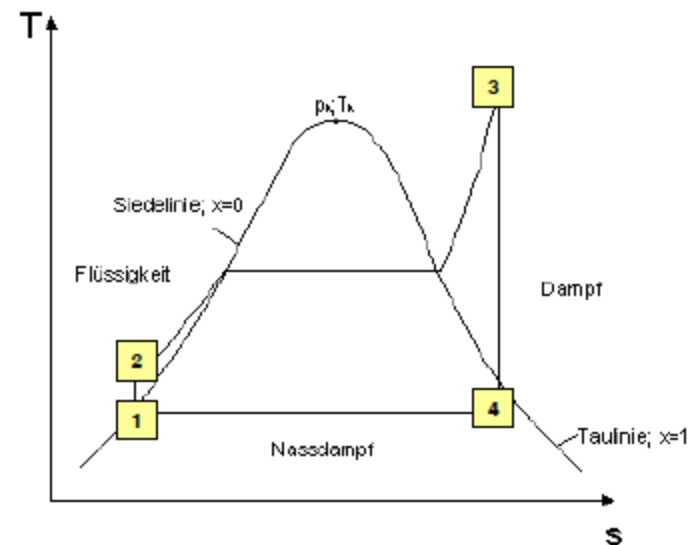
T-s-Diagramm
