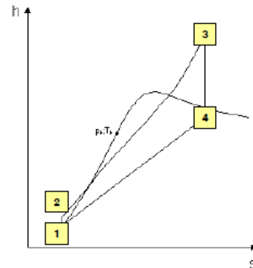
h-s-Diagramm
