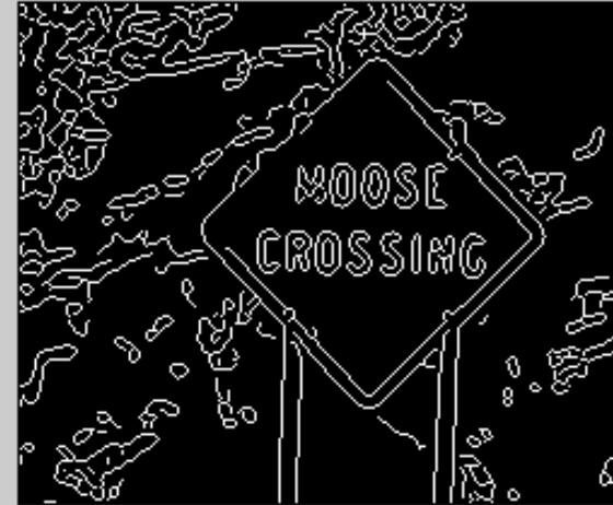
Canny Edge
