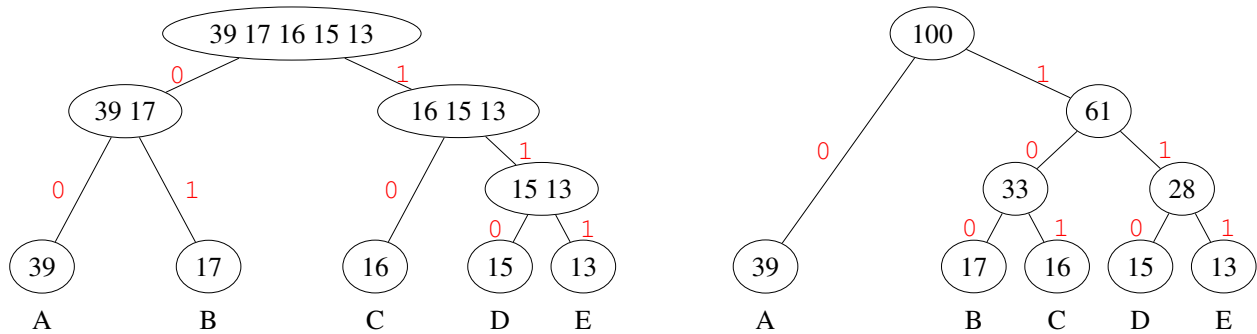
FIGURE 1 – à gauche : code de Shannon-Fano ; à droite : code de Huffman
