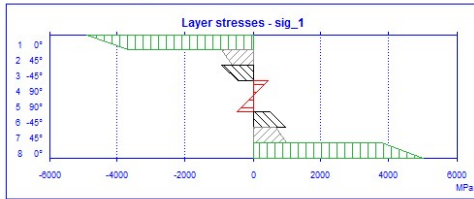
Actual stress, Actual (=Eq) strain
