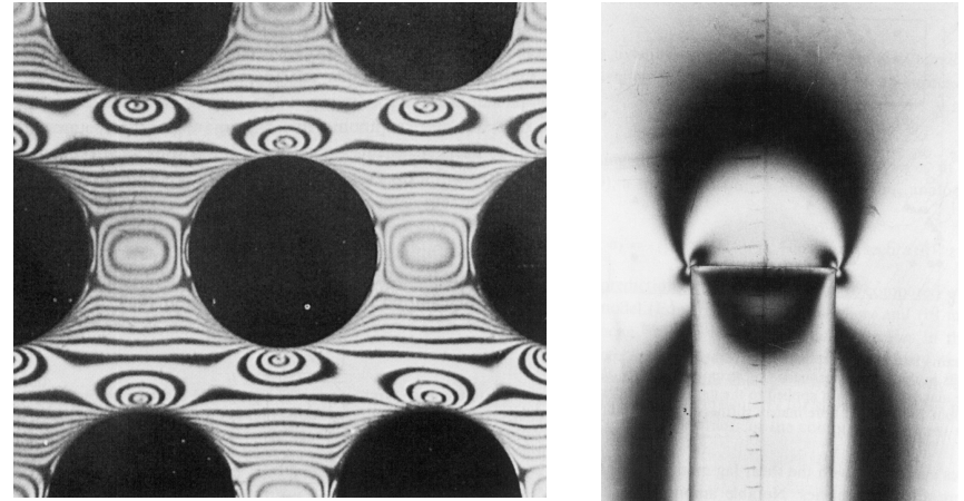
Visualisation des isochromes (lignes d'isocontraintes) dans une matrice polymère enrobant des fibres
