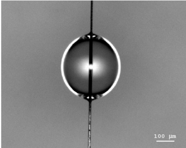
Résine époxy sur fibre de carbone
